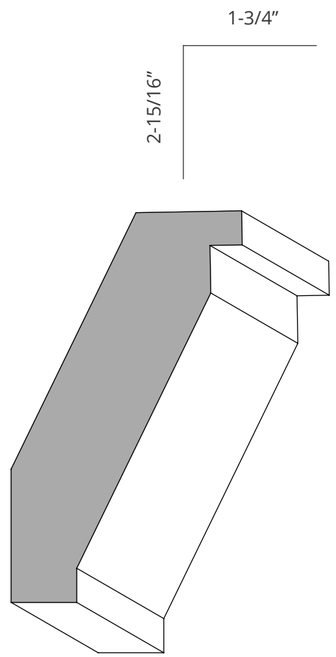
CR525 7/8" x 3-3/8"
